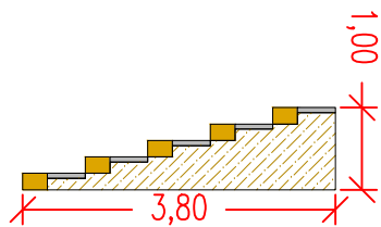
ŘEZ SCHODIŠTĚM č.1 5stupňů 0,2x0,3x1,6m
