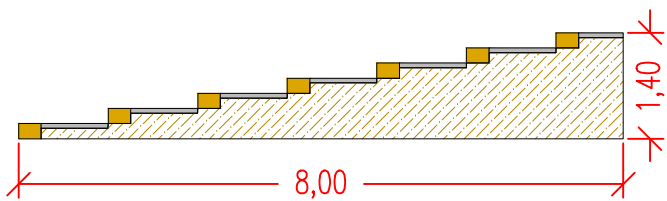
ŘEZ SCHODIŠTĚM č.2 7stupňů 0,2x0,3x1,2m
